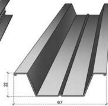
Hat Furring Channel
